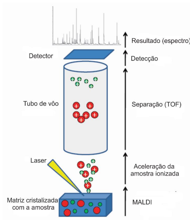
Figura 2- Princípios da espectrometria de massas por (MALDI-TOF MS)
