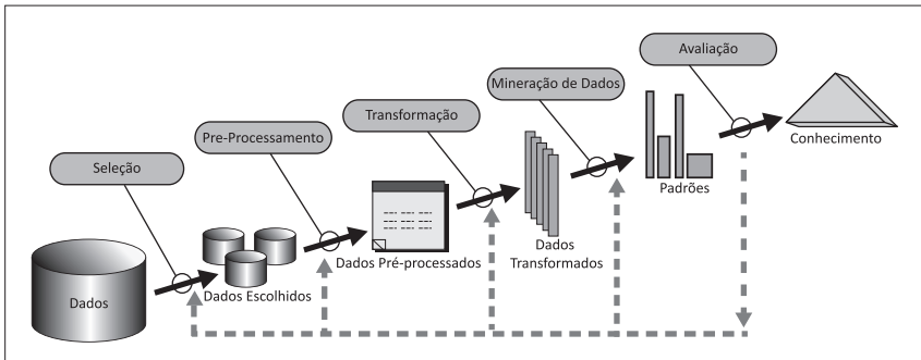
FIGURA 1 – Processo KDD
