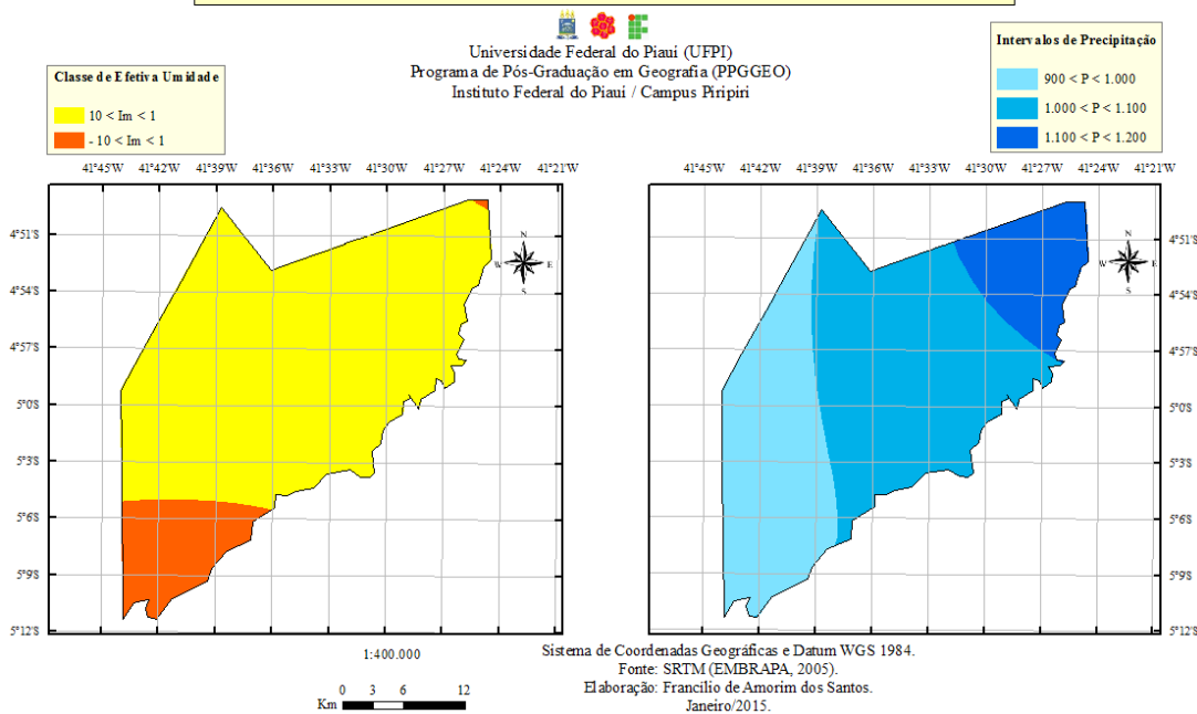
Figura 4. Índice efetivo de umidade e precipitação anual média de Juazeiro do Piauí.
