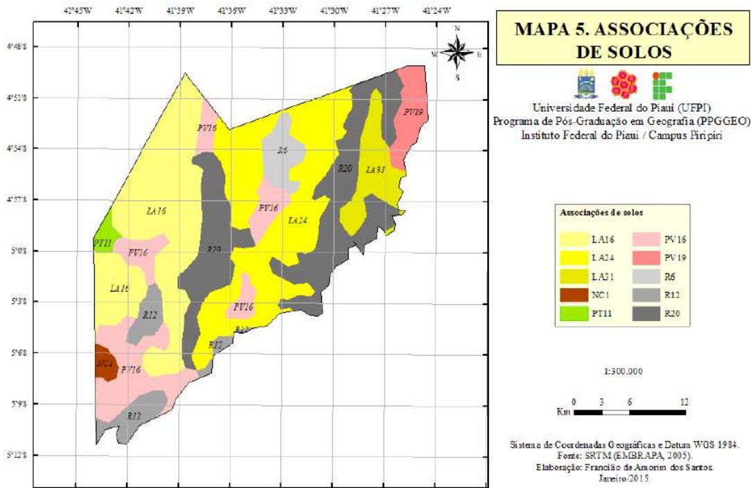
Figura 5. Esboço das associações de solos do município de Juazeiro do Piauí.
