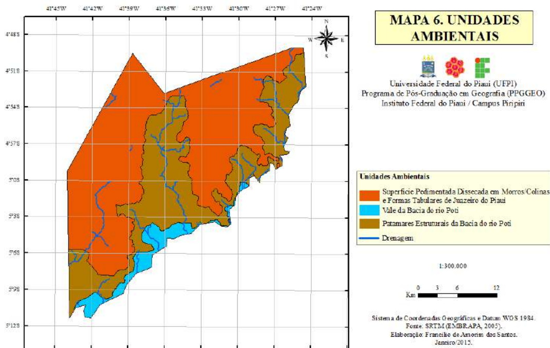
Figura 6. Unidades geoambientais mapeadas no município de Juazeiro do Piauí.
