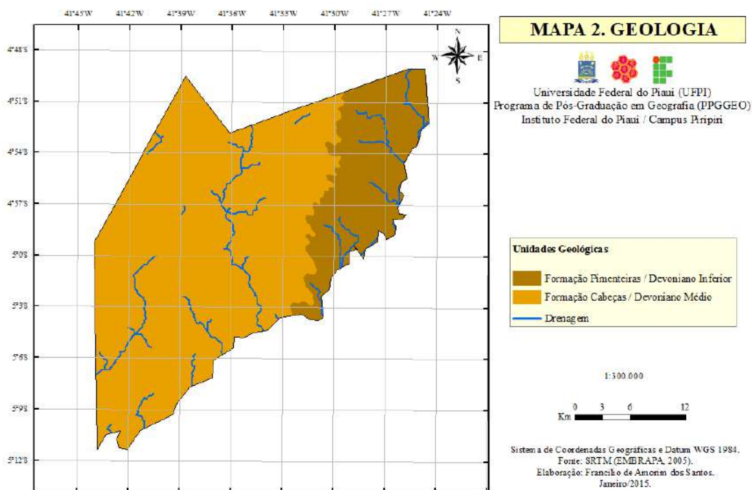
Figura 2. Esboço das formações geológicas do município de Juazeiro do Piauí.
