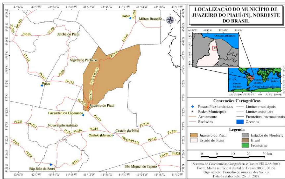
Figura 1. Localização do município de Juazeiro do Piauí, setor nordeste do estado do Piauí.
