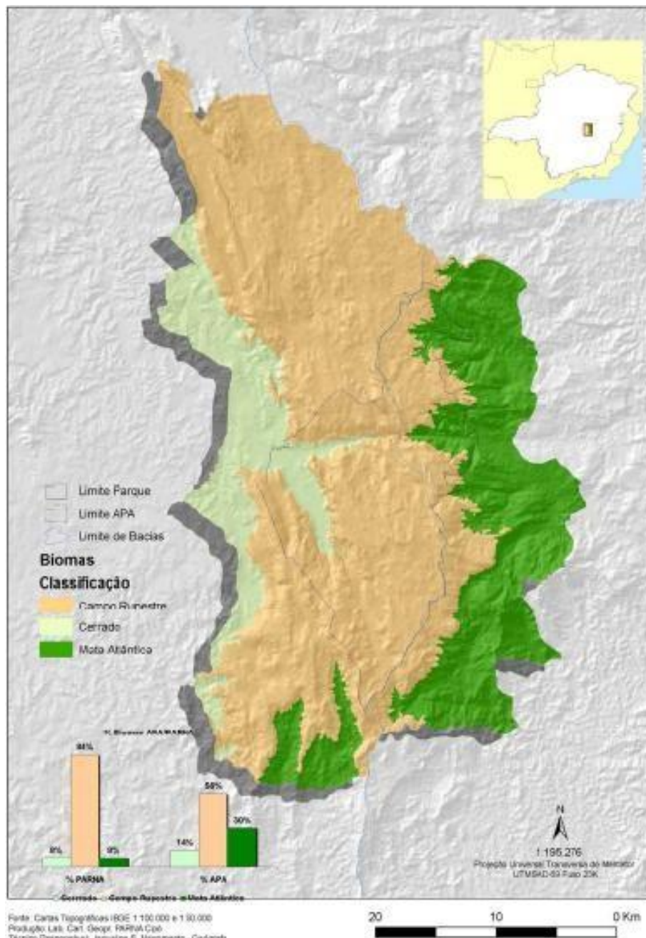
Figura 5: Principais Fitofisionomias encontradas na Serra do Cipó
