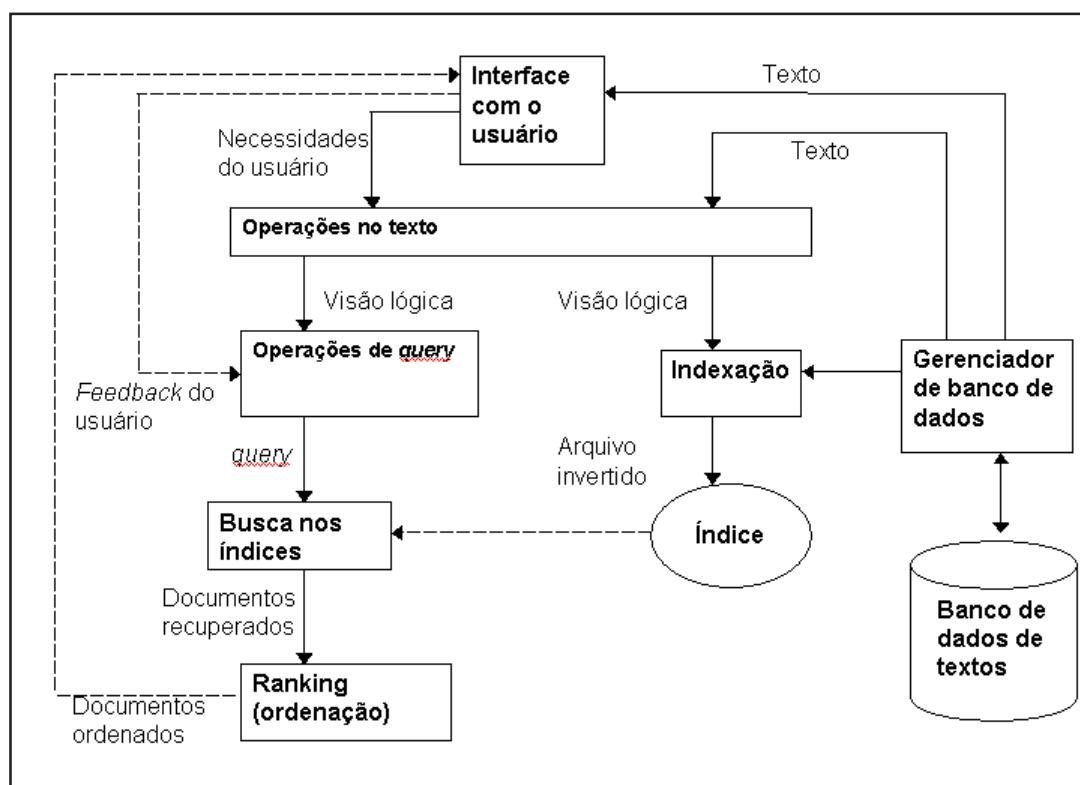
FIGURA 1 – O processo de recuperação de informações (adaptado de BAEZA-YATES e RIBEIRO-NETO, 1999, p. 10).
