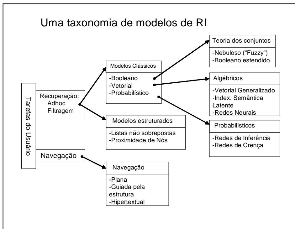
FIGURA 2 – Uma taxonomia de modelos de RI (adaptado de BAEZA-YATES e RIBEIRO-NETO, 1999, p. 21).
