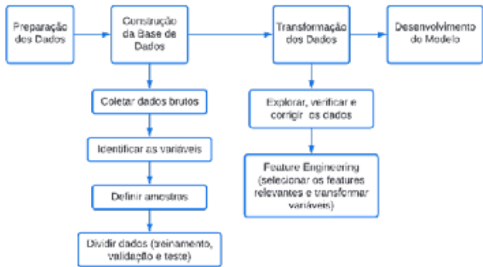
Figura 1 - Fluxograma da preparação de dados Fonte: Adaptado pelo Autor (Google AI, 2023).
